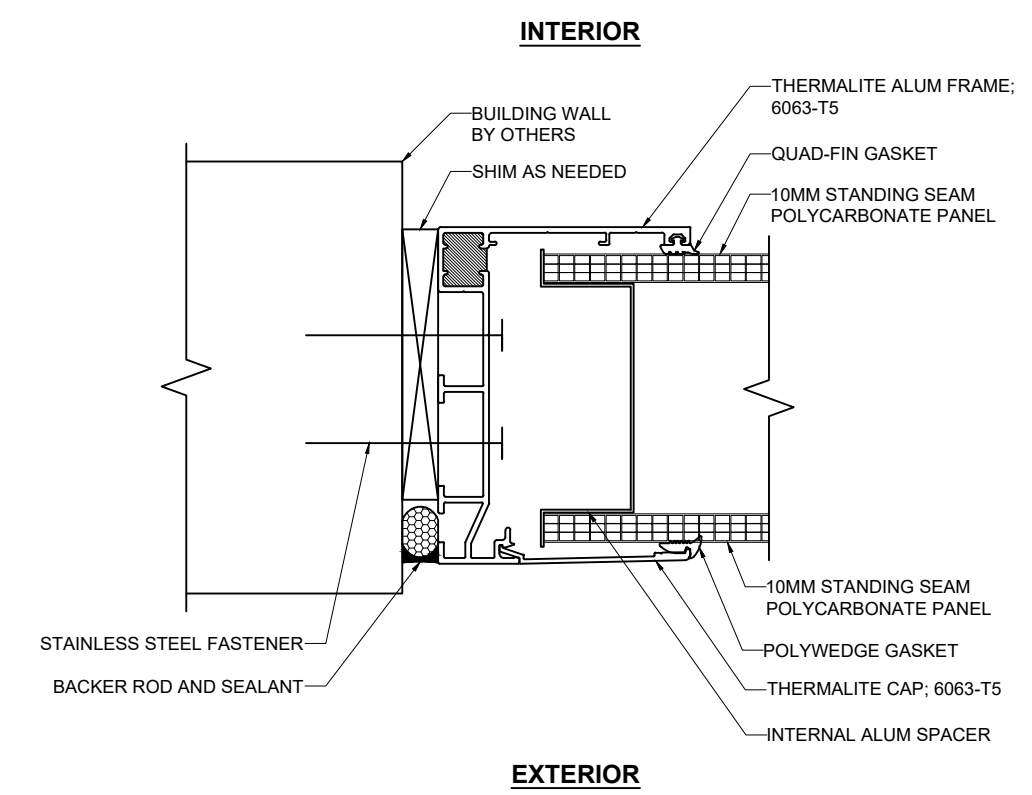
F 1 JAMB SCALE: 3/8" = 1"
