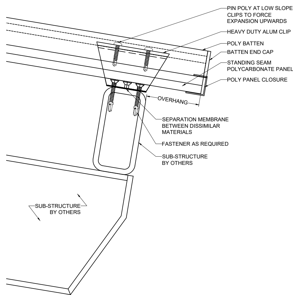
E 1 BASE SCALE: 3/8" = 1"
