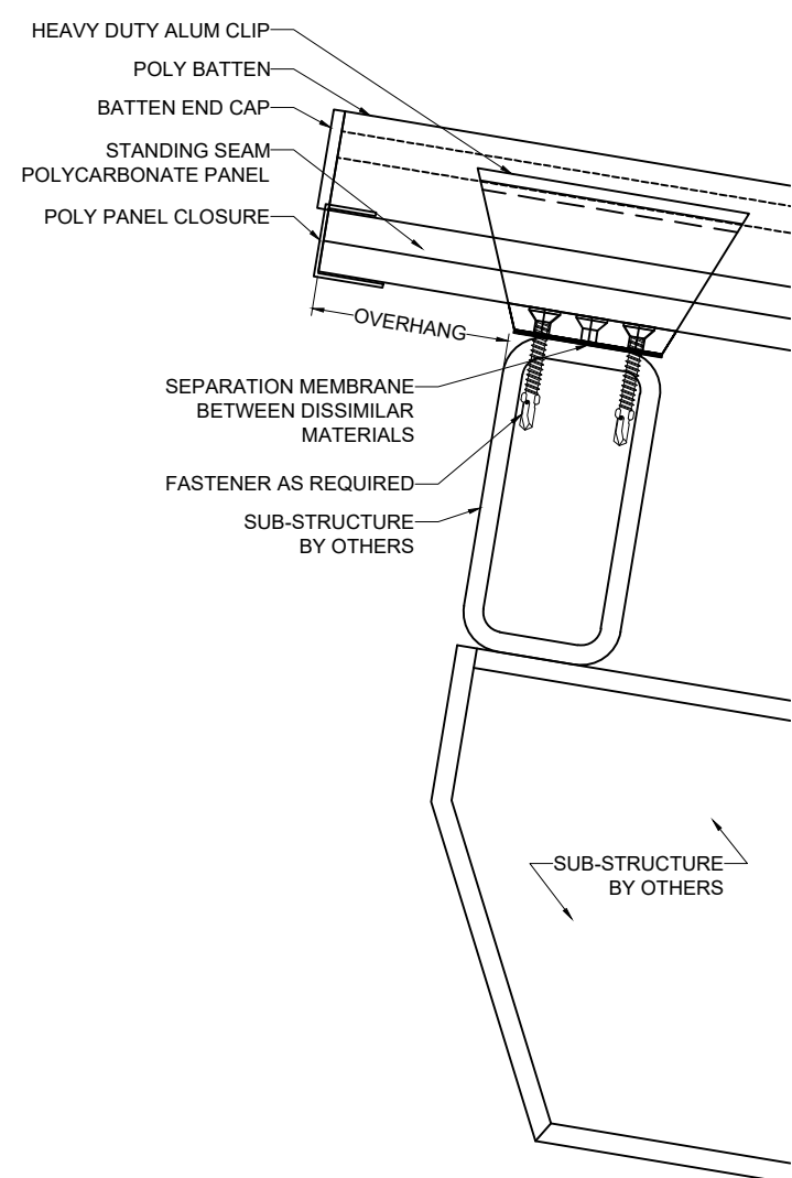
C 1 HEAD SCALE: 3/8" = 1"
