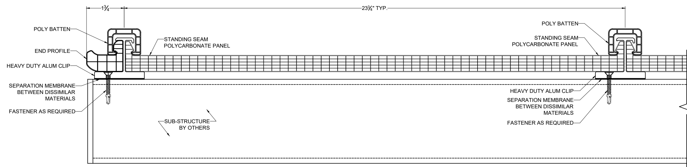
F 1 END SCALE: 3/8" = 1"
