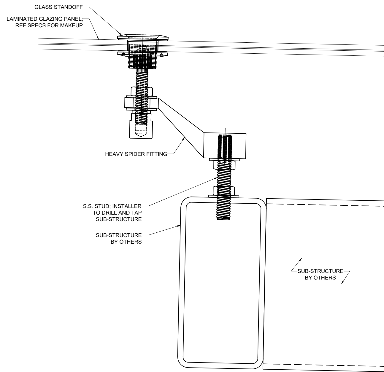
C 1 HEAD SCALE: 3/8" = 1"
