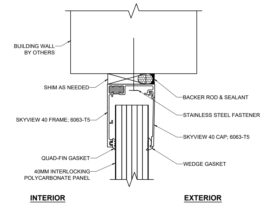
D 1 HEAD SCALE: 3/8" = 1"
