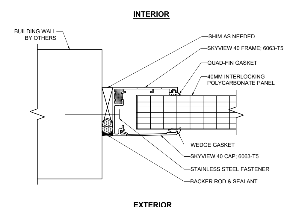
F 1 JAMB SCALE: 3/8" = 1"
