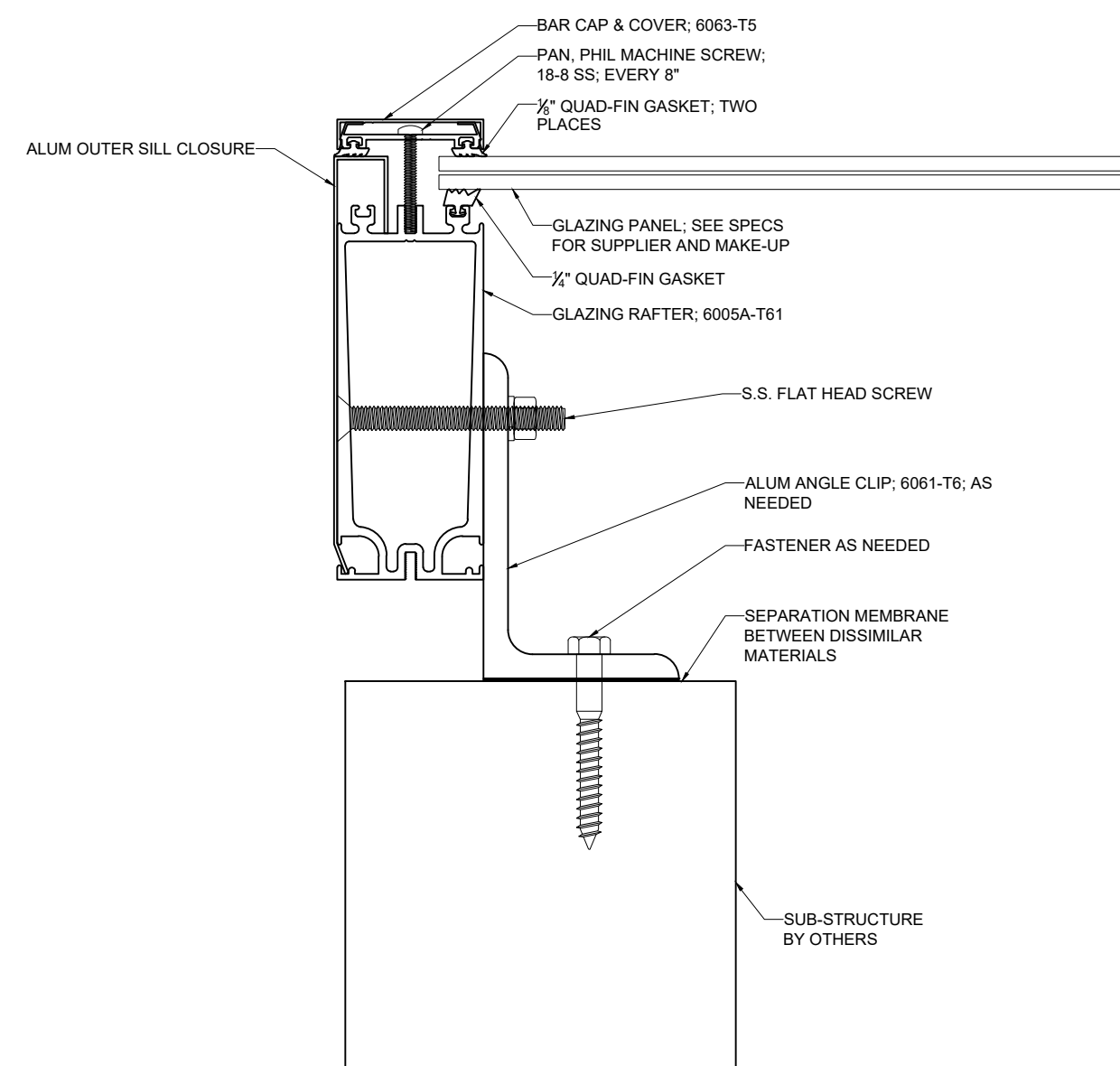
E 1 GABLE SILL/RAFTER SCALE: 3/8" = 1"
