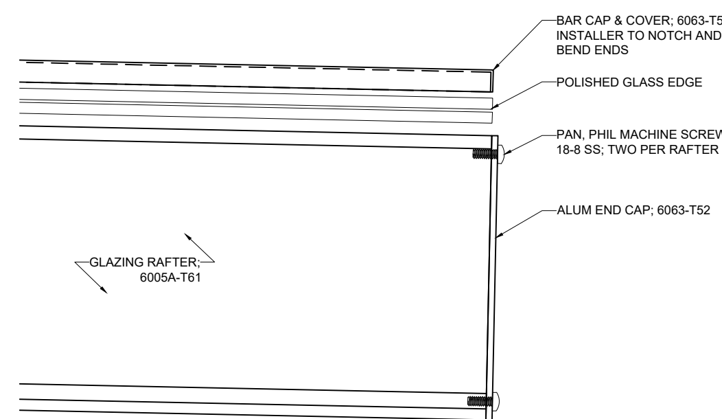
D 1 BASE HEAD SIM. SCALE: 3/8" = 1"
