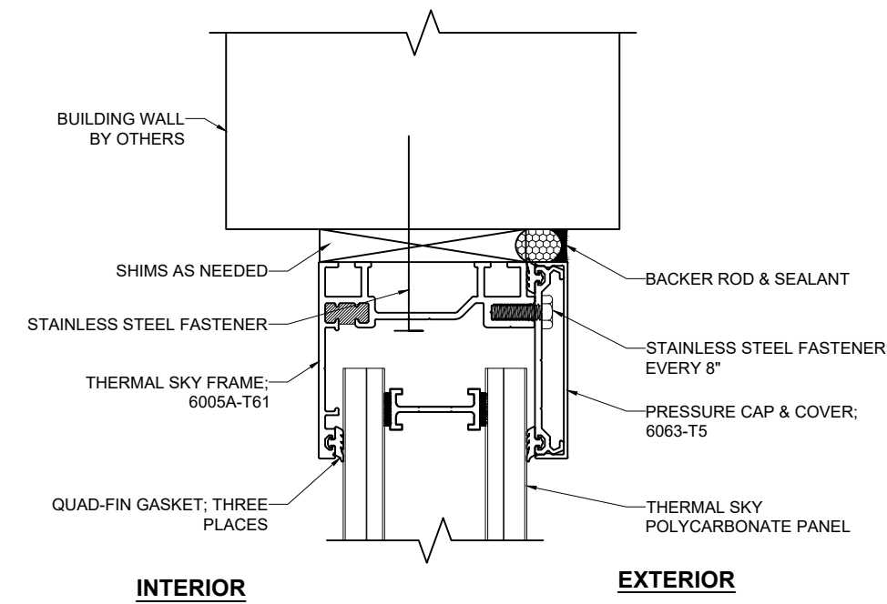
D 1 HEAD SCALE: 3/8" = 1"
