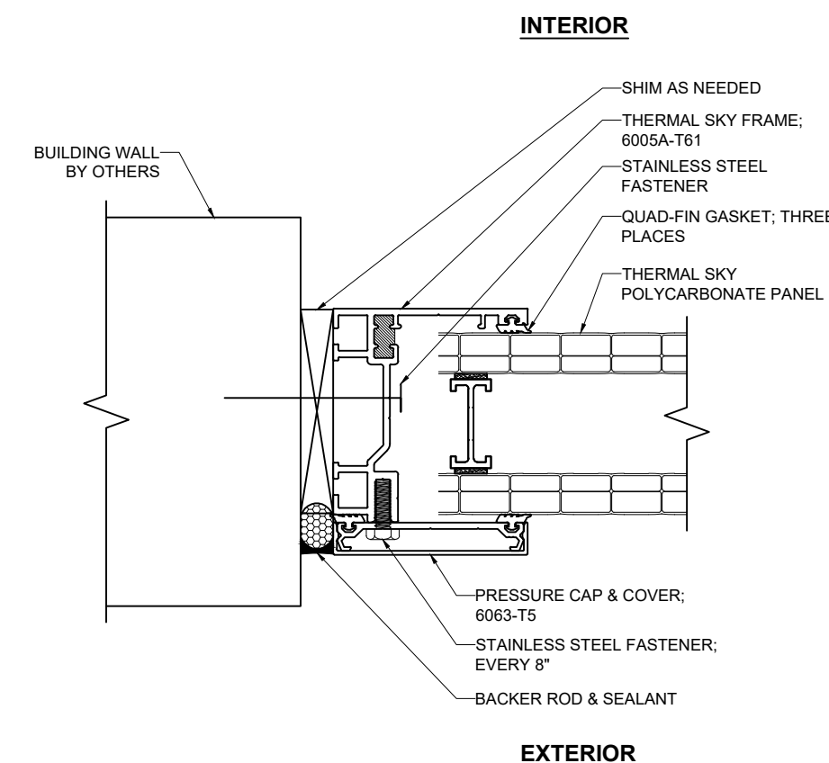
F 1 JAMB SCALE: 3/8" = 1"
