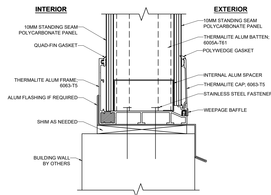
E 1 BASE SCALE: 3/8" = 1"
