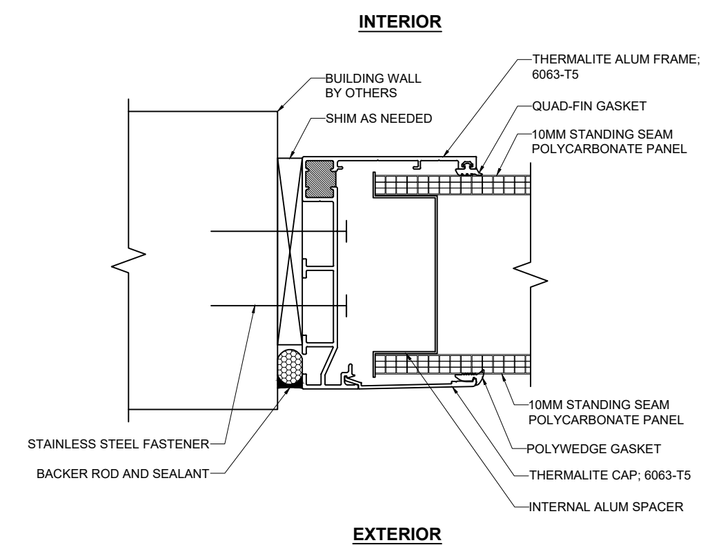
F 1 JAMB SCALE: 3/8" = 1"
